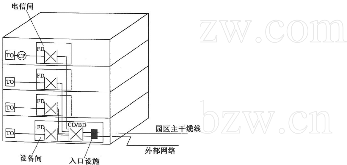
图 1 综合布线配线设备典型设置
